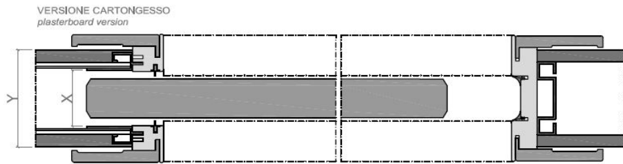
SEZIONE ORIZZONTALE horizontal section
