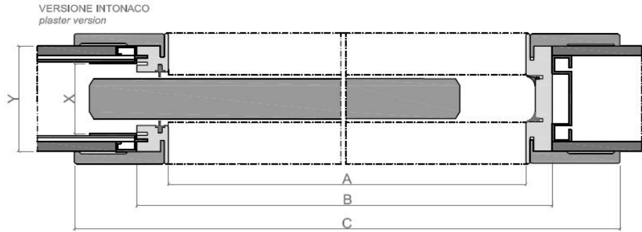
SEZIONE ORIZZONTALE horizontal section
