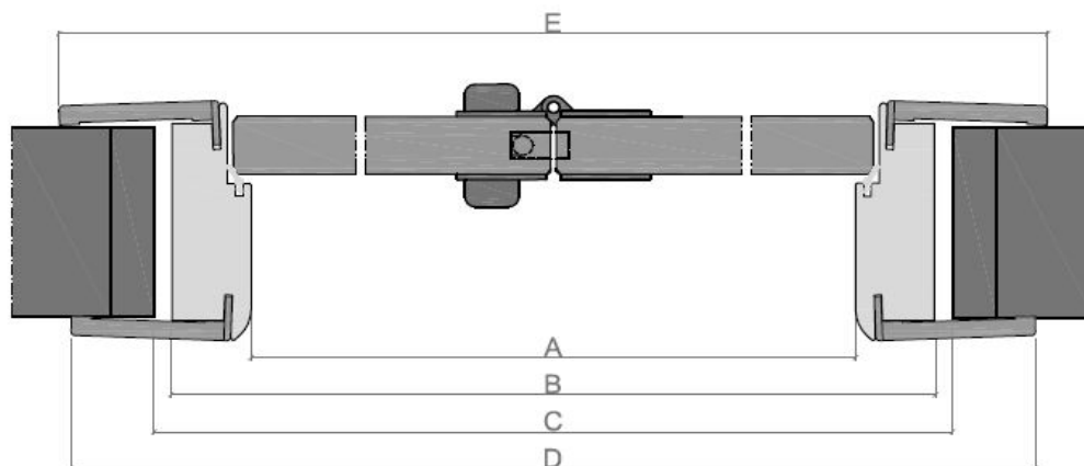
SEZIONE ORIZZONTALE horizontal section
