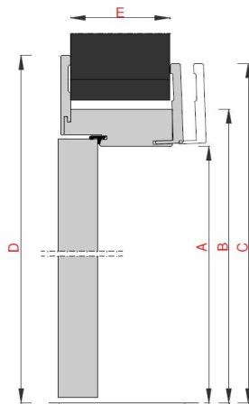
SEZIONE VERTICALE
