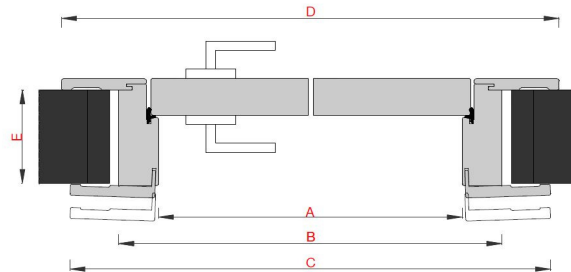
SEZIONE ORIZZONTALE
