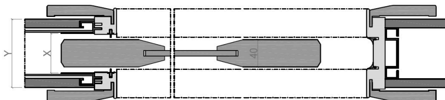
SEZIONE ORIZZONTALE horizontal section
