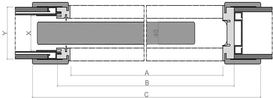
VERSIONE CARTONGESSO plasterboard version
