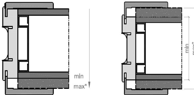
CONTROTELAIO DECENTRATO metallic subframe decentralized
