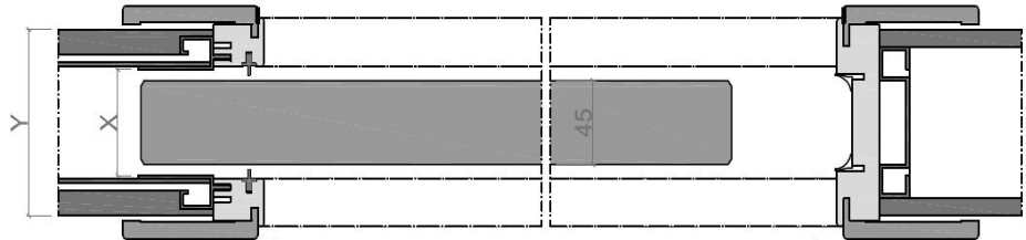
DIMENSIONI CONTROTELAIO / MURO dimensions metallic subframe / wall
